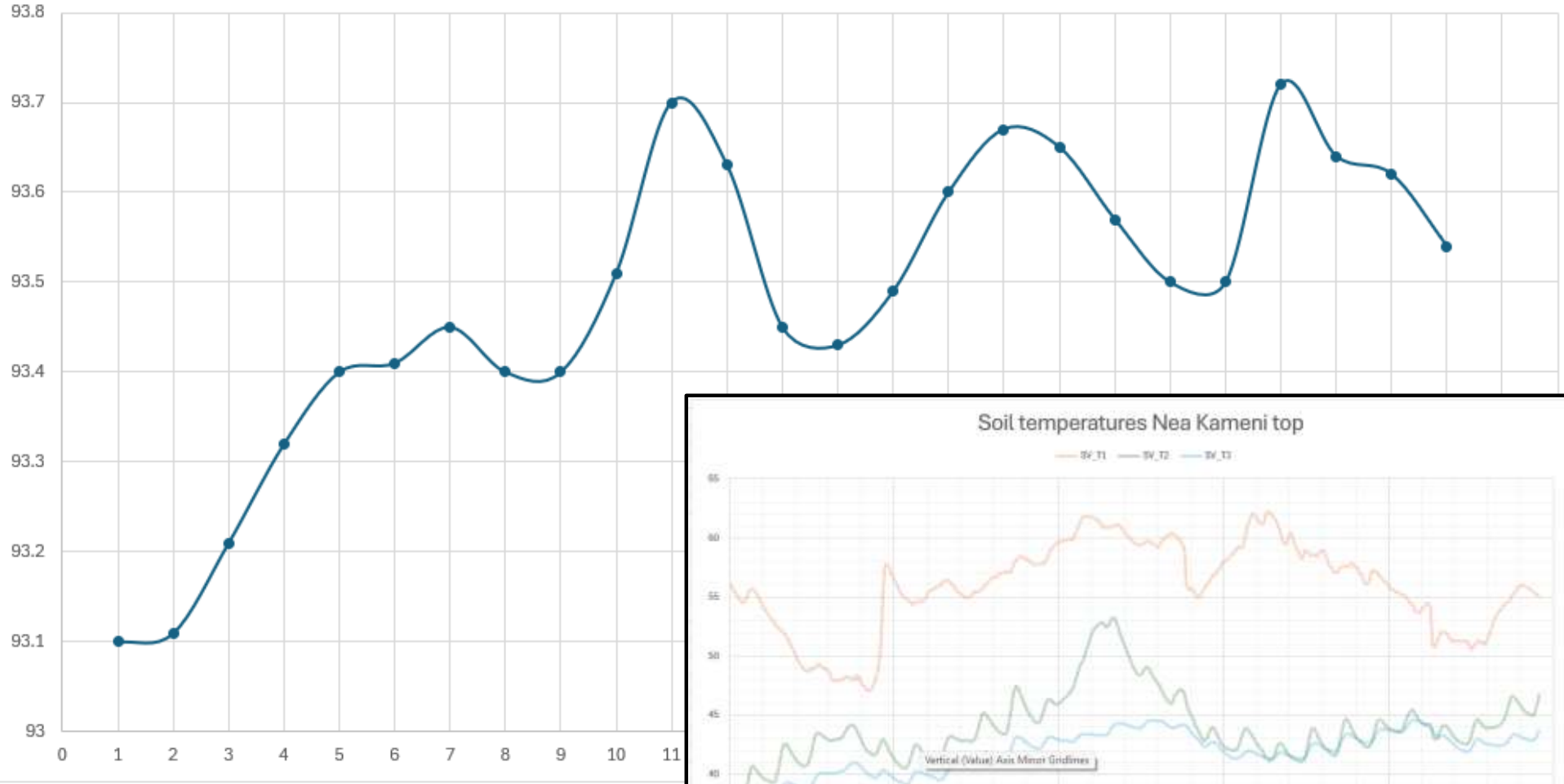
Θερμοκρασία Ατμίδας Ν.Καμένης (ΕΑΓΜΕ) – ΙΑΝ 2025
